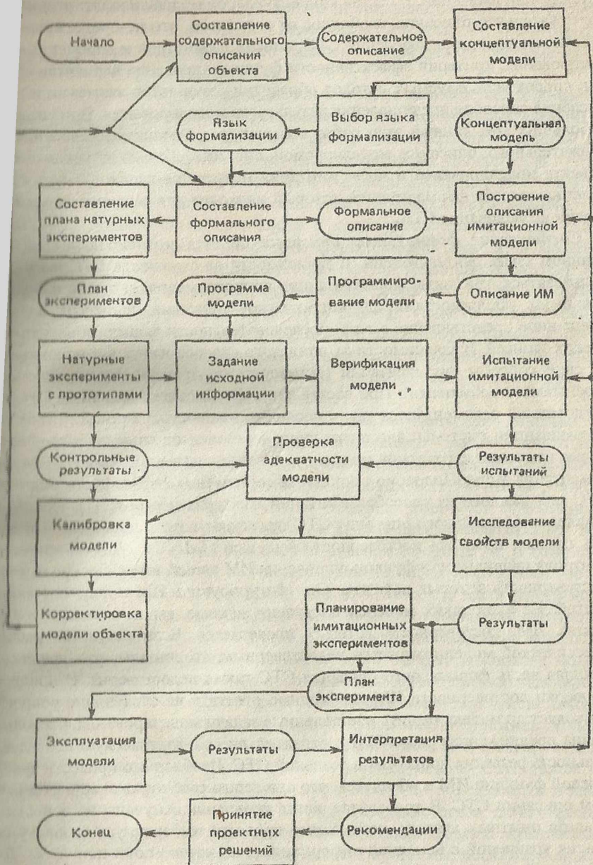
Рис. 1.7. Схема взаимосвязи технологических этапов имитационного моделирования ТС
