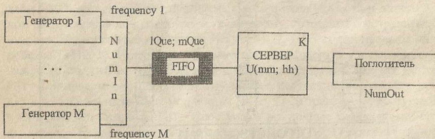
Рис. 7.4. Граф-схема модели простейшей системы массового обслуживания.
