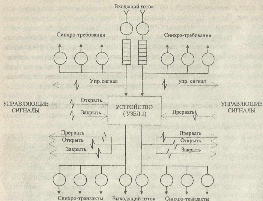
Рис. 4.1. Обобщенный узел сети СМО
