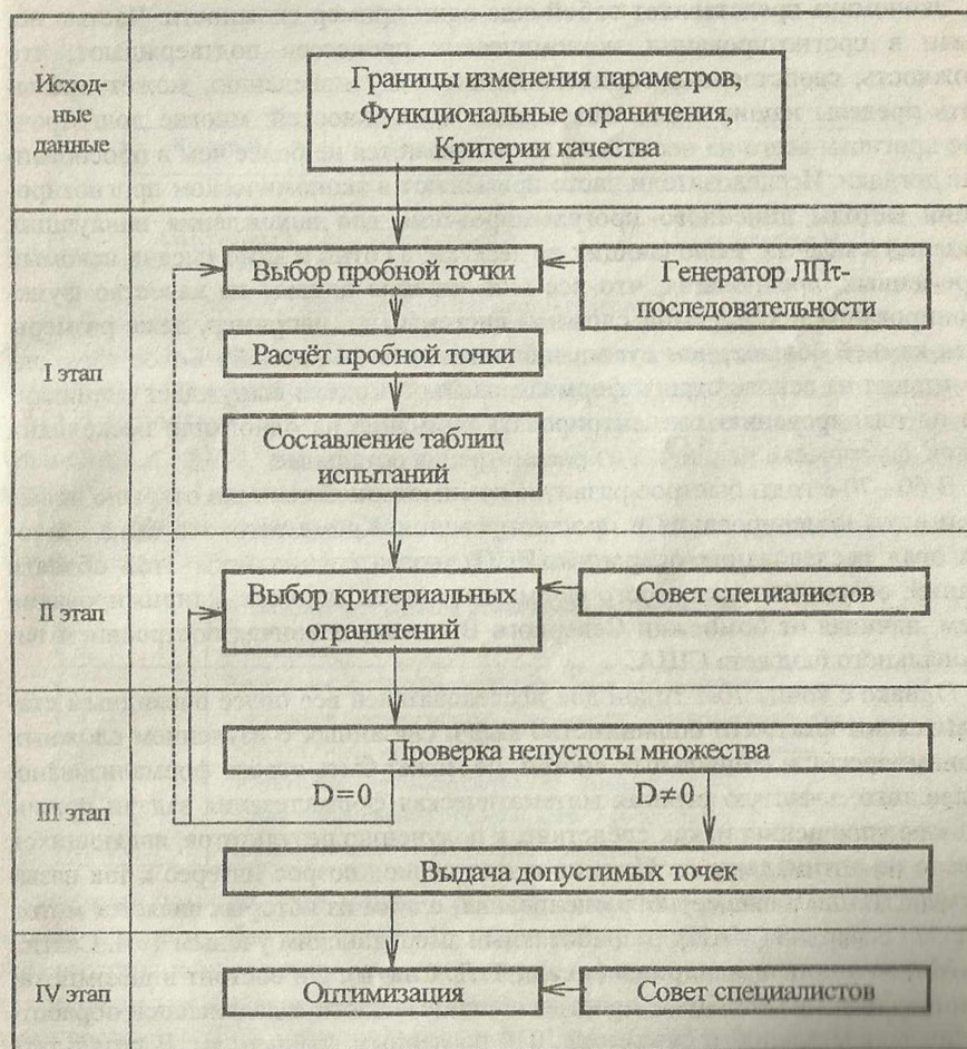
Рис. 6.3. Схема диалогового алгоритма метода ЛПГ-последовательности
