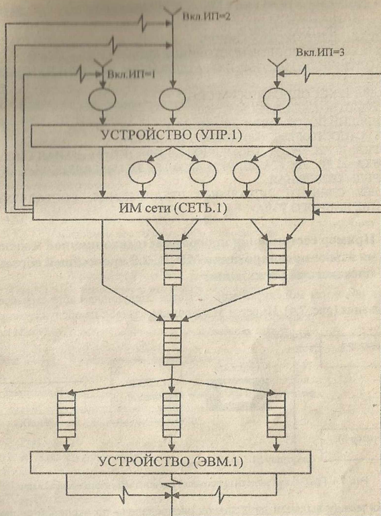
Рис. 7.3. Фрагмент модели СМО с управляемыми источниками
