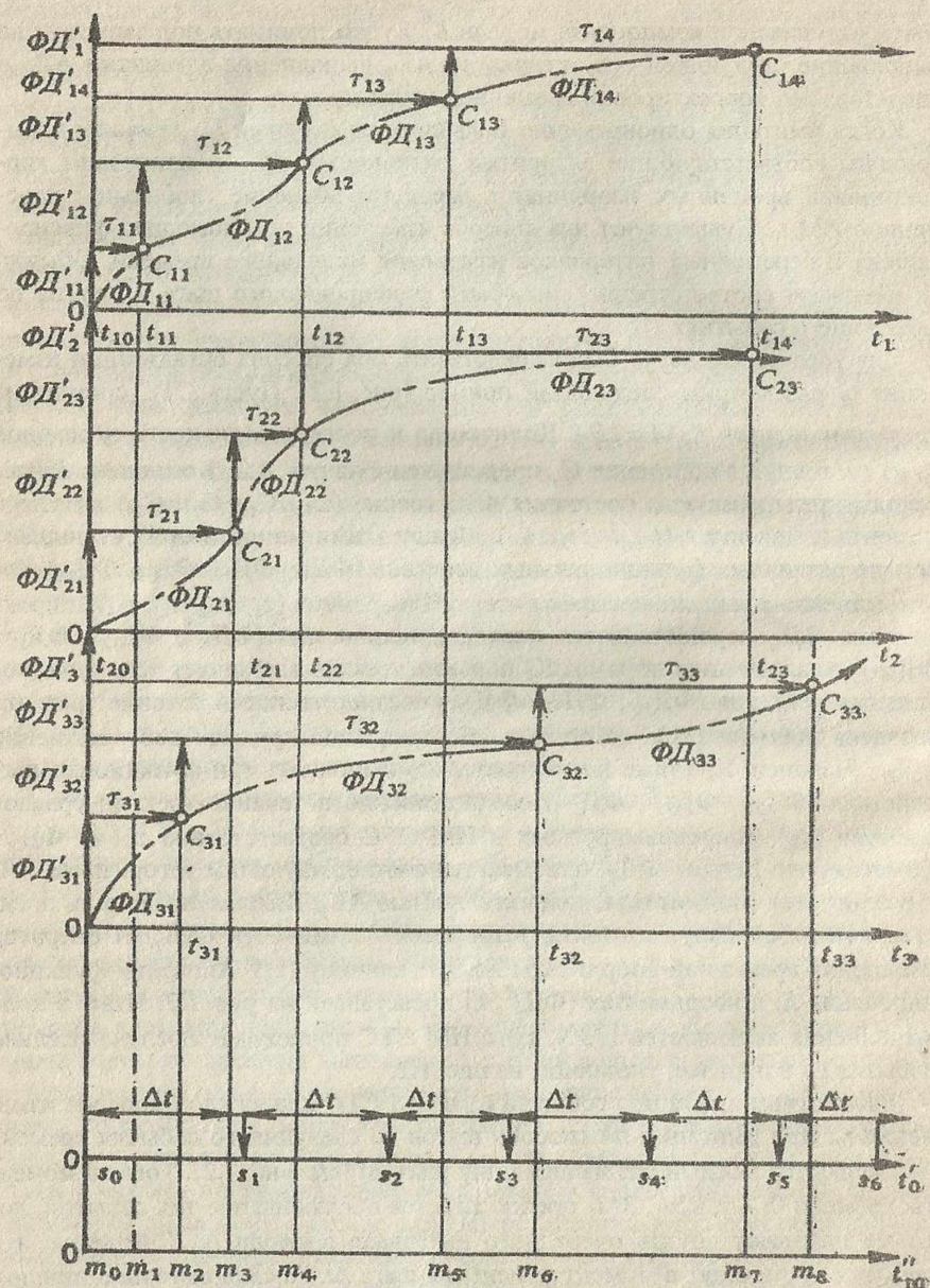
Рис. 1.2. Временная диаграмма имитационного моделирования событий в реальной системе из трех компонент
