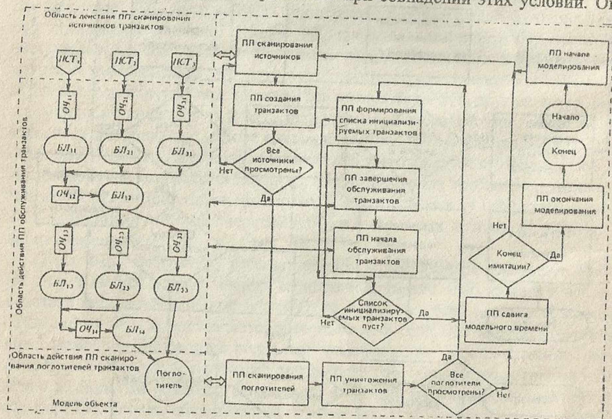
Рис. 1.5. Схема взаимодействия управляющей программы с моделью объекта при транзактном способе имитации
