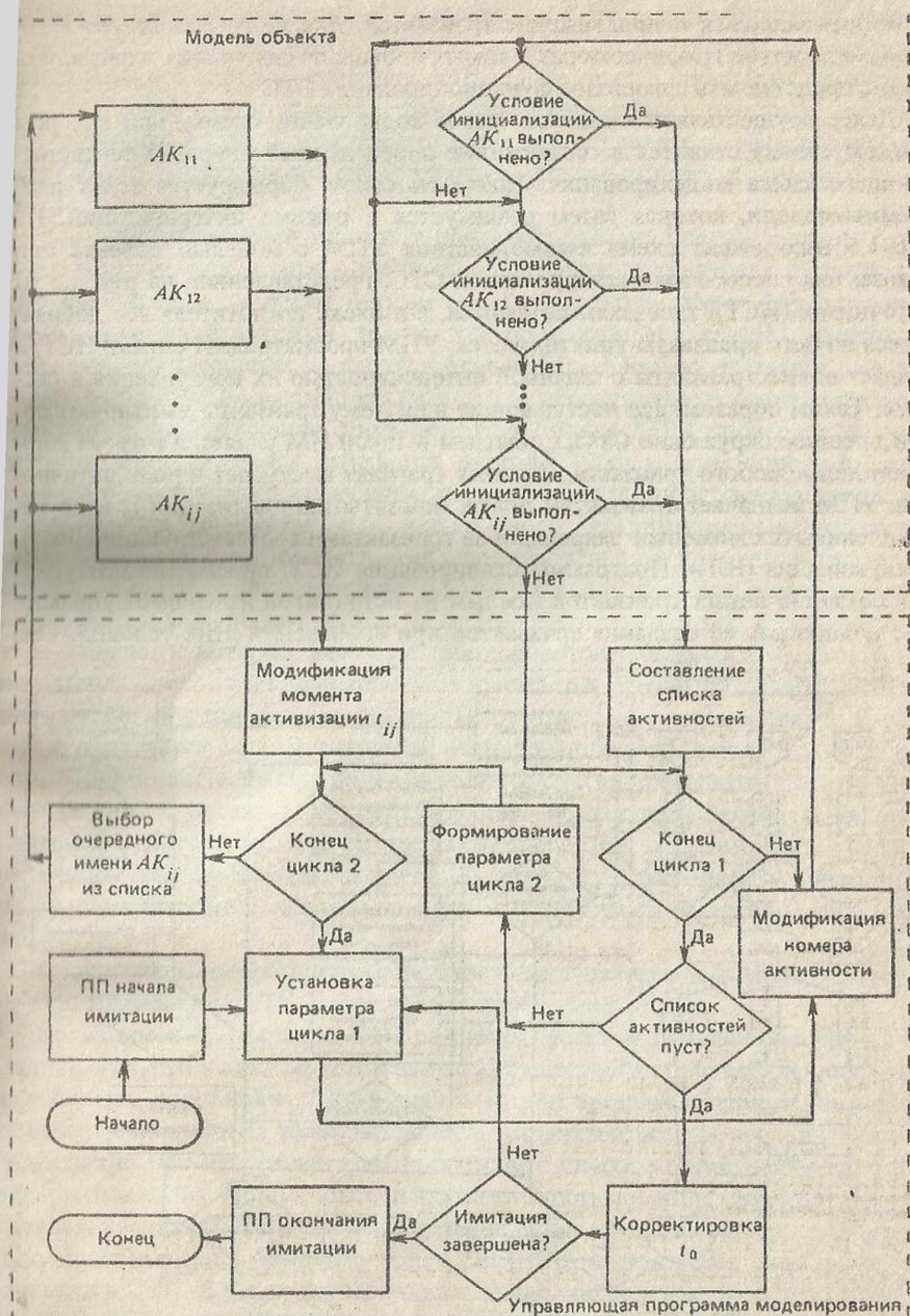
Рис. 1.4. Схема модели объекта, состоящей из активностей
